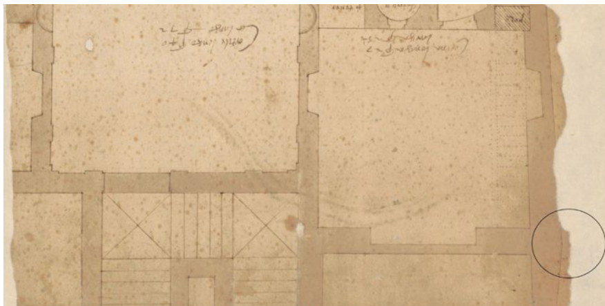
Figura 11. Francesco Paciotto (attr.), progetto per il retro di palazzo Torres-Lancellotti, dettaglio del quarto angolo su via della Cuccagna, disegno su carta, 1548-1550 circa. Roma, Archivio di Stato di Roma, Ospedale di San Giacomo degli Incurabili, b. 1505, 1/92.
